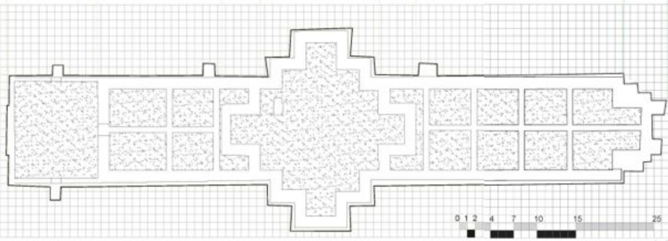
แบบแปลนวัดบ้านดอน อำเภอเมือง จังหวัดสุพรรณบุรี
