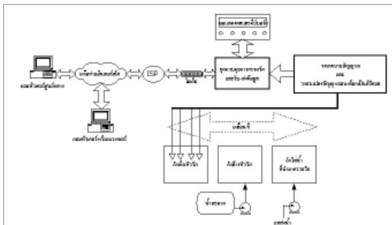
รูปที่ 1 Block Diagram ของชุดควบคุมการตรวจวัดคุณภาพสิ่งแวดล้อม
