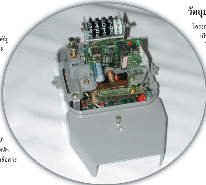
รูปแสดงมิเตอร์ไฟฟ้าซึ่งได้ติดตั้ง Reading Module เข้าไปแล้ว
